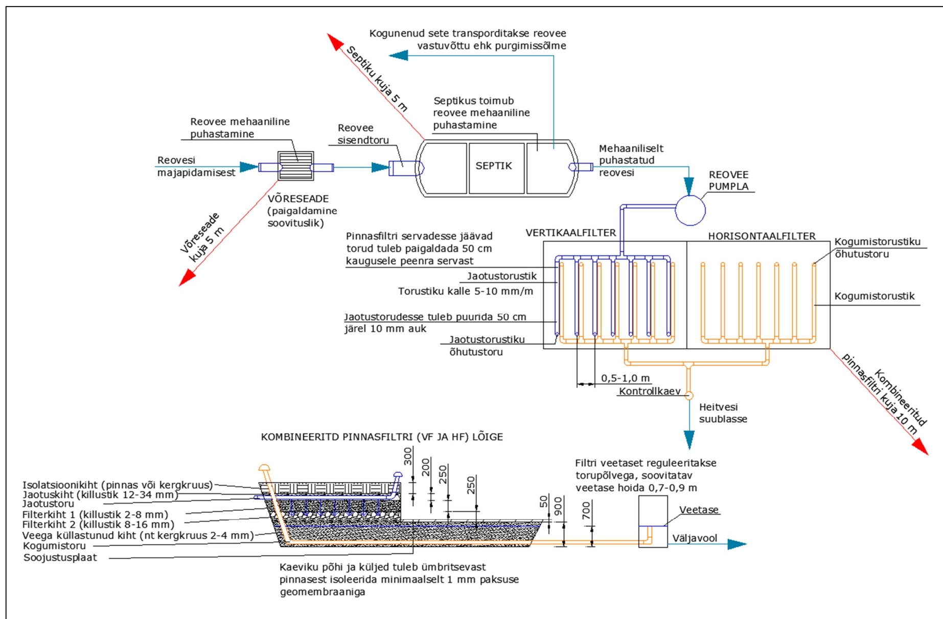
Joonis 11. Kombineeritud pinnasfiltersüsteemist koosneva reoveepuhastussüsteemi tehnoloogiline skeem [19].
