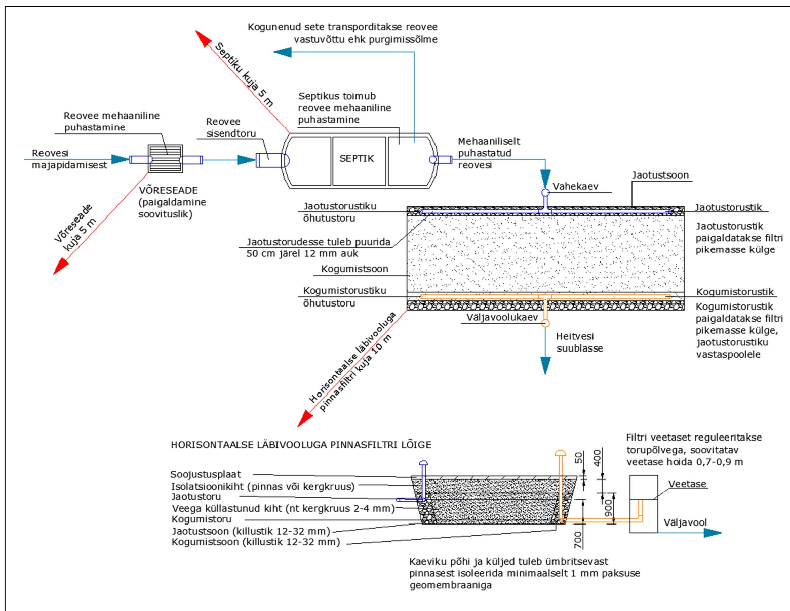
Joonis 10. Horisontaalse läbivooluga pinnafiltrist koosneva reoveepuhastussüsteemi tehnoloogiline skeem [19].
